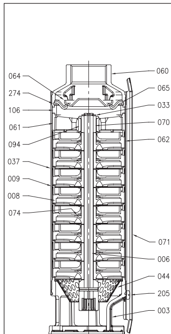
ВИД В РАЗРЕЗЕ, WINNER 4N1-4N2-4N4
