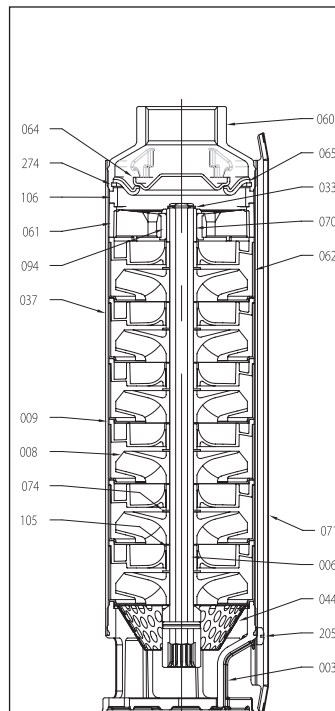
ВИД В РАЗРЕЗЕ, WINNER 4N7
