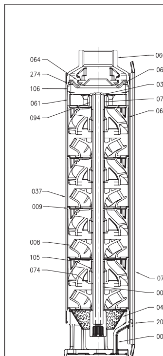
ВИД В РАЗРЕЗЕ, WINNER 4N15
