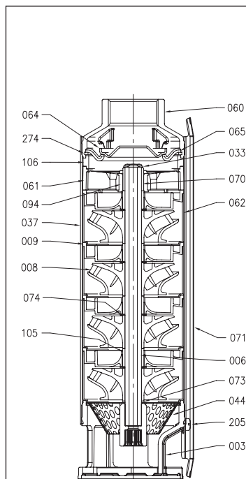
ВИД В РАЗРЕЗЕ, WINNER 4N10
