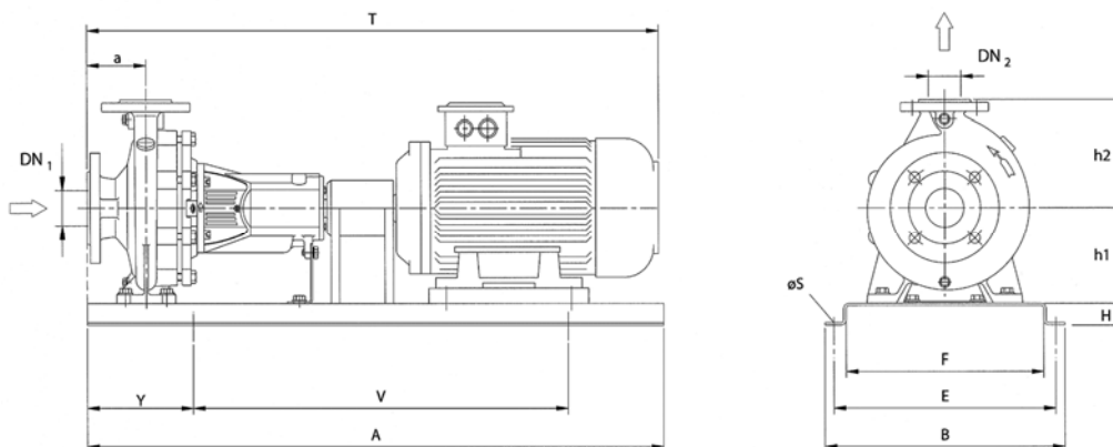
Dimension table 32 - 40 - 50
