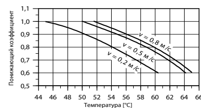
Обмотка РЕ2/РА, 5,5–37 кВт
